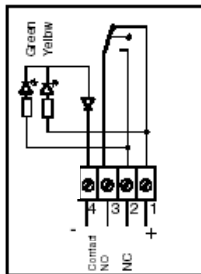
Anschlußplan mechanische Endschalter Stellung OFFEN
